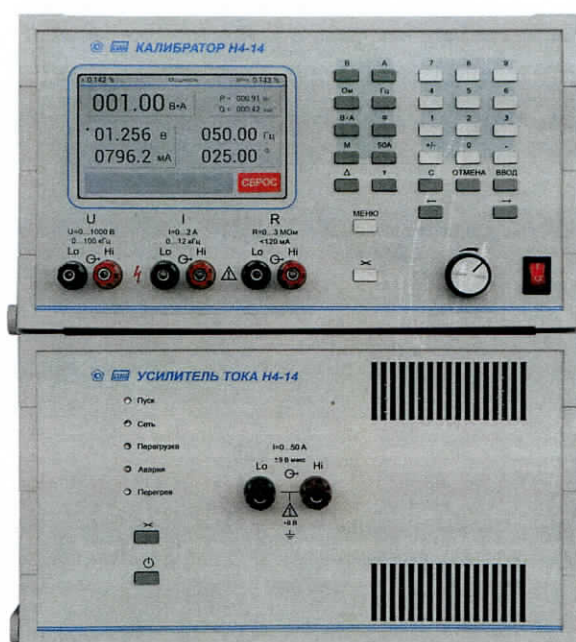
Рисунок 1 – Общий вид калибратора
