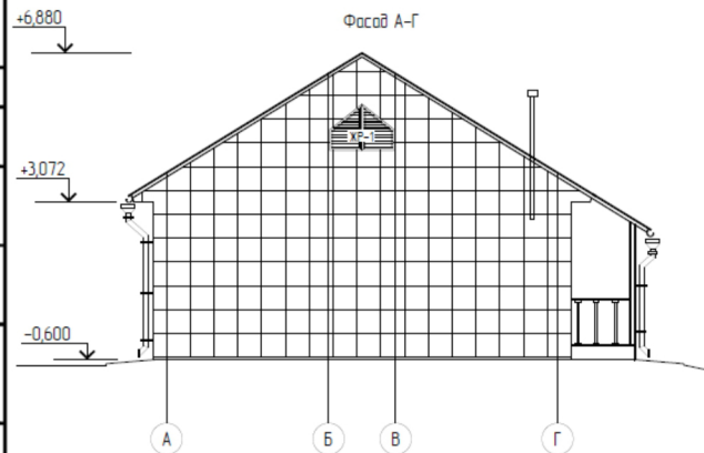
Фасад А-Г
