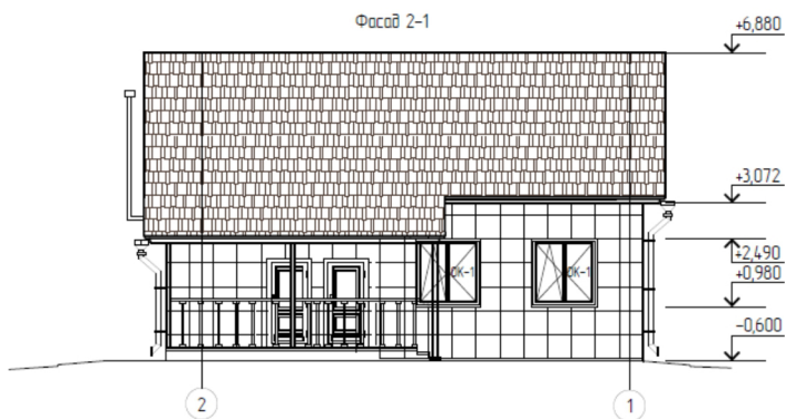
Фасад 2-1
